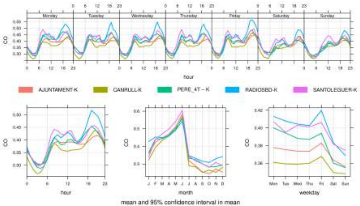
Figura 5: Variació temporal del CO.
