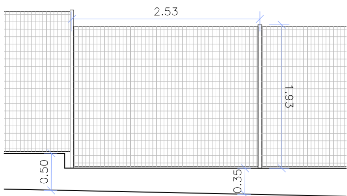
S1-13ut Tanca perimetral sobre muret de bloc de formigó.
